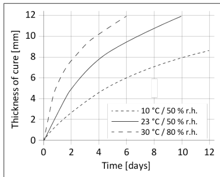
Διάγραμμα 1: Ταχύτητα ωρίμανσης SikaTack® Panel
