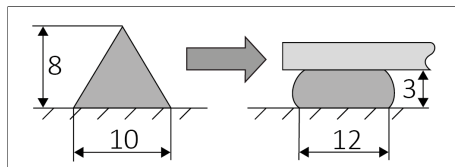
Σχήμα 1: Συνιστώμενη διαμόρφωση κορδονιού
