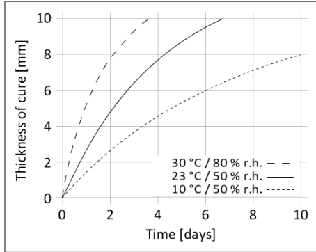
Διάγραμμα 1: Ταχύτητα ωρίμανσης Sikaflex®-268
