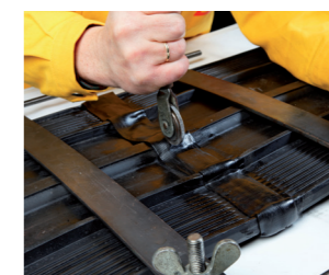
Εφαρμογή ταινίας κάλυψης, πίεση και των δύο ταινιών κάλυψης.
