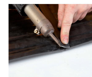
Ενίσχυση με ταινία συγκόλλησης χρησιμοποιώντας πιστόλι θερμού αέρα
