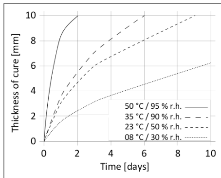
Διάγραμμα 1: Ταχύτητα ωρίμανσης Sikasil® AS-70
