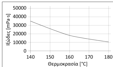
Διάγραμμα 1: Το ιξώδες σε συνάρτηση με τη θερμοκρασία. Κατά τη διακοπή εργασιών, το SikaMelt®-230 πρέπει να επεξεργαστεί ως ακολούθως:
