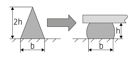
Σχήμα 1: Συνιστώμενη μορφή κορδονιού εφαρμογής
